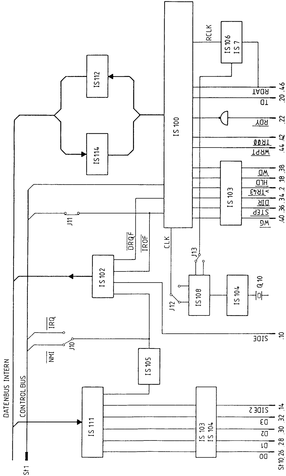
Bild 10: Blockschaltbild Floppy-Disk-Controller
